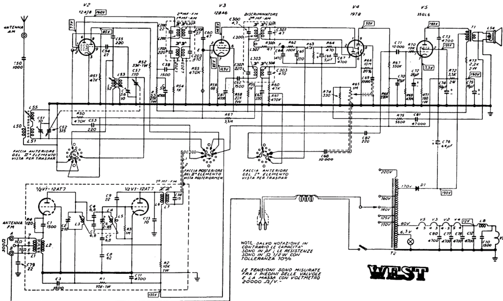
WEST RADIO-TV - Mod. MIKE. Apparecchio AM/FM, con gamma onde medie da 525 a 1610 kc/s, e banda onde ultracorte da 87,3 a 100,5 Mc/s. Media frequenza AM a 455 kc/s, MF/FM a 10,7 Mc/s. Resa d'uscita 2 watt. Consumo 36 watt.
